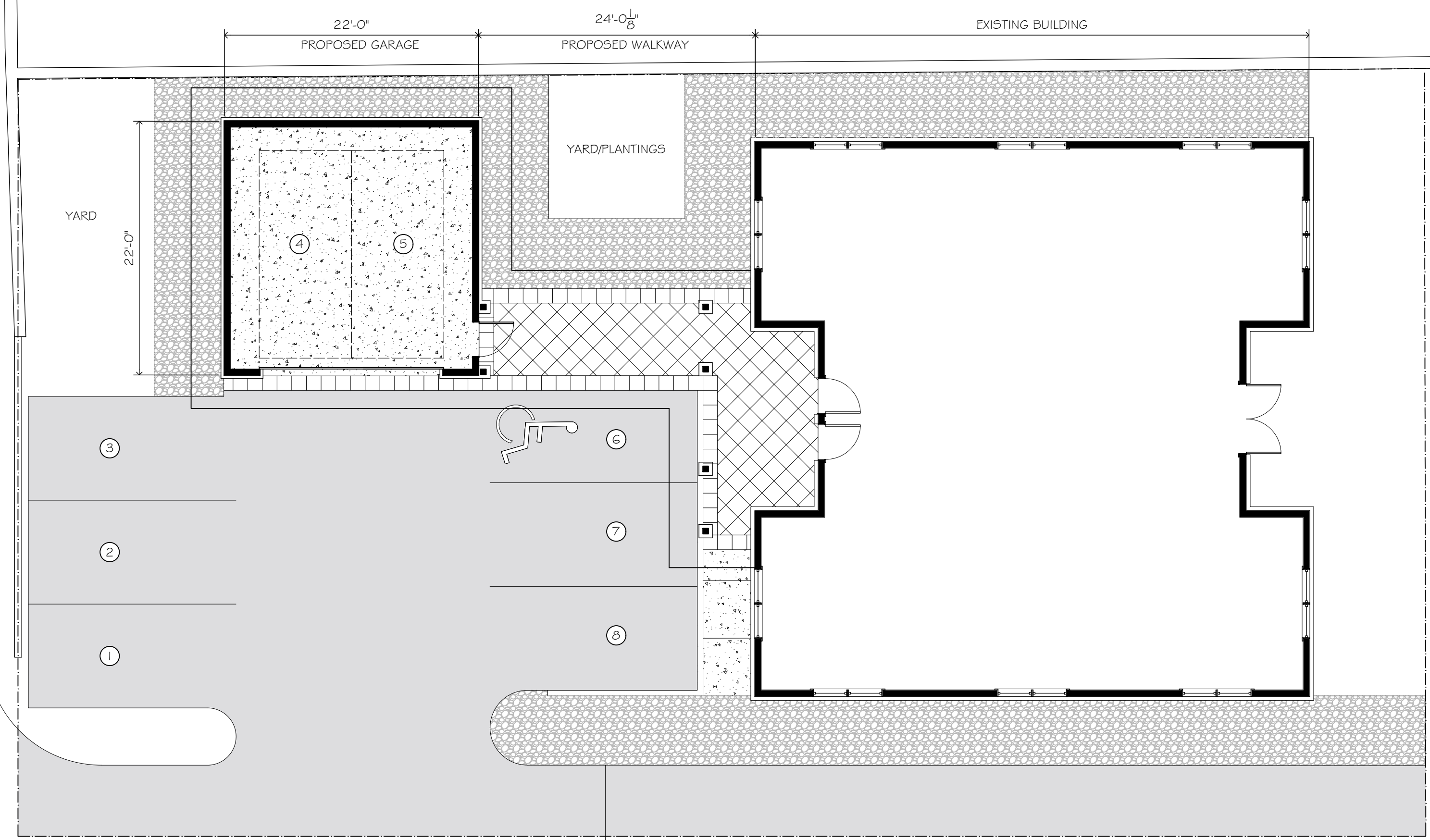
1 SITE PLAN 1/8"=1'-0"
